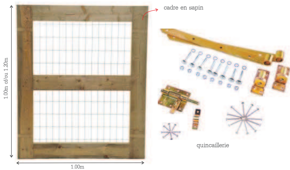
gonds et ferrures de la photo jusqu'au épuisement de stock, ce modèle part après
