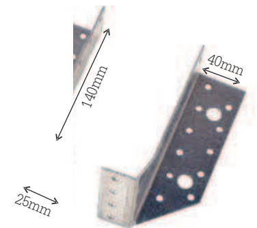
support à écartement variable
