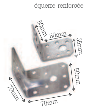
attache en L
